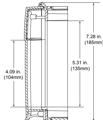
Du Montage En Surface Vue Latérale (Entretoise De 32 mm)
