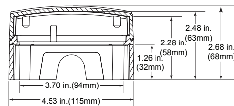
Vue Du Dessus (Entretoise De 32 mm)
