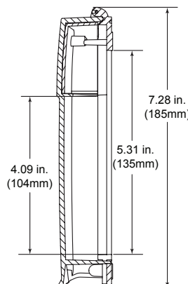
Du Montage Encastré Vue Latérale
