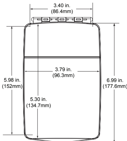
Du Montage Encastré Vue Avant
