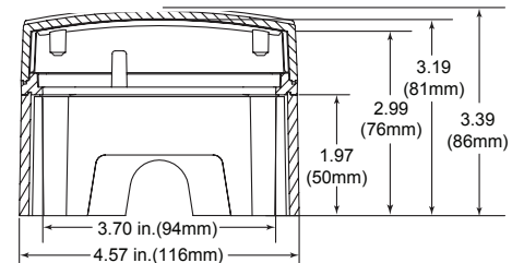
Vue Du Dessus (entretoise de 50 mm) lorsque le STI-6507 est acheté
