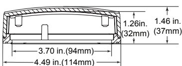
Du Montage Encastré Vue Latérale
