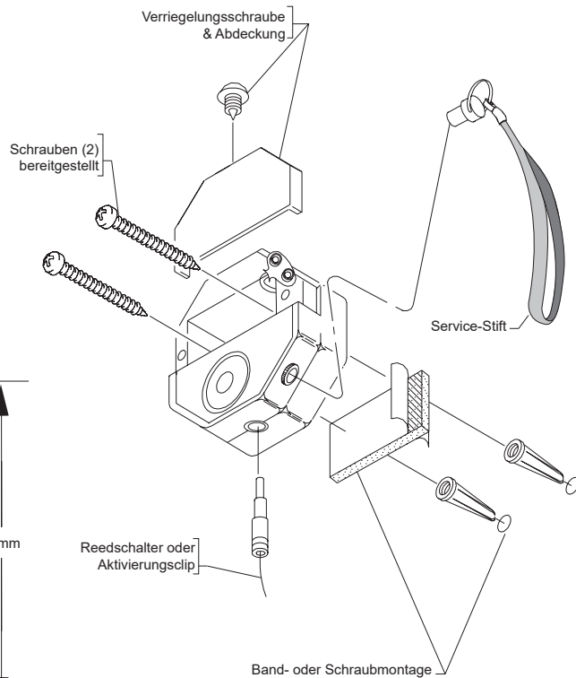
Magnetischer Reedschalter
