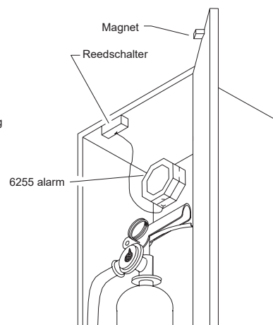
Magnetische Reedschalter-Aktivierung
