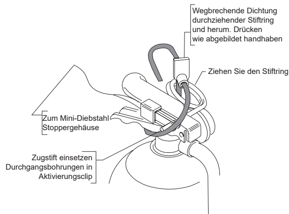
Stahl-Kontaktklammer Schalteraktivierung
