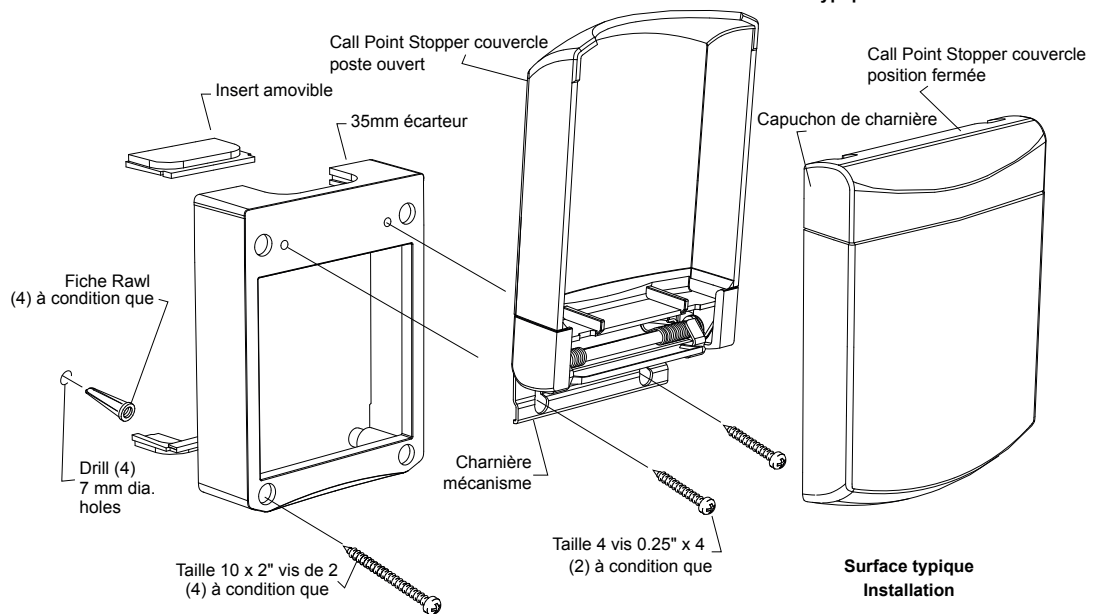
Montage affleurant typique
