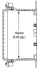
SECCIÓN A-A
