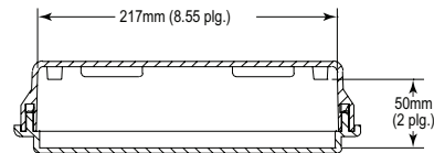
SECCIÓN B-B
