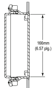
SECCIÓN A-A
