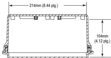
SECCIÓN B-B
