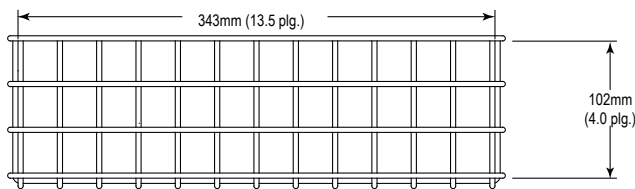
VISTA SUPERIOR EN PLANTA
