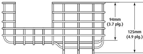
STI-9720 VISTA SUPERIOR
